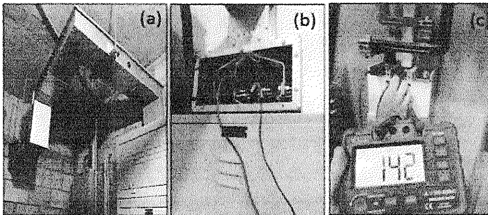
Figura 12: Ensaio de resistência de isolamento em barramento blindado (a) na entrada principal do sistema do barramento blindado "Flange de entrada" (b), utilizando-se Megôhmetro digital(c).
